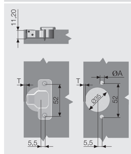
Карта сверления под чашку 52 мм
