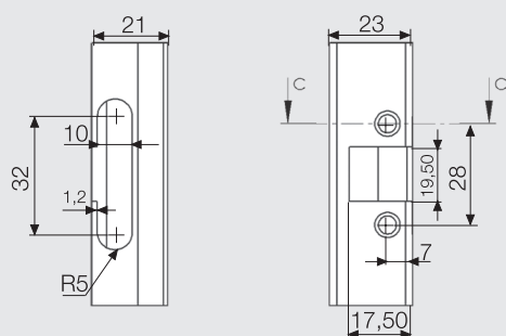
Сечение C-C
