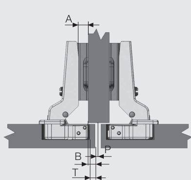
A - Монтажная планка
