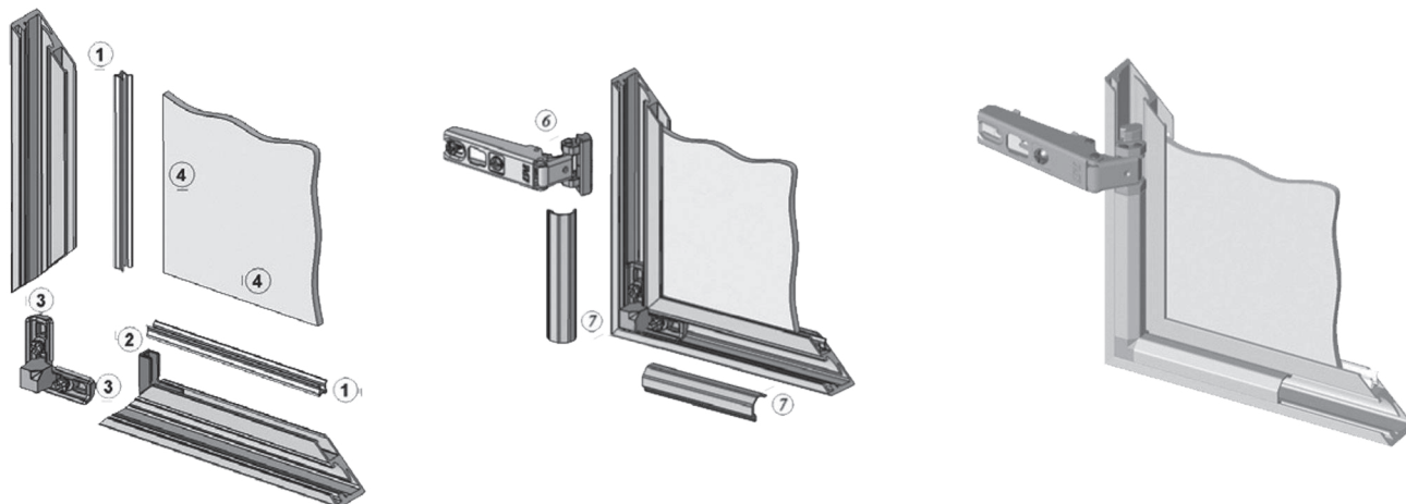
Угловое соединение
