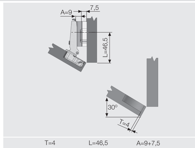
Карта сверления под чашку 48 мм
