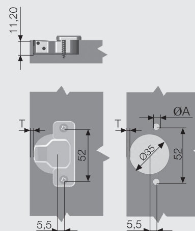
Карта сверления под чашку 52 мм
