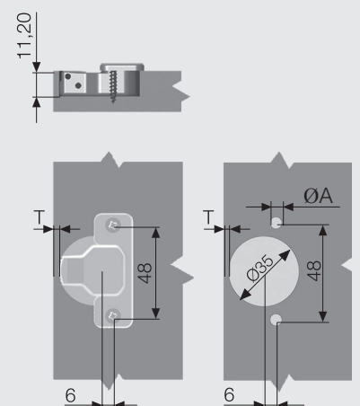
Карта сверления под чашку 48 мм
