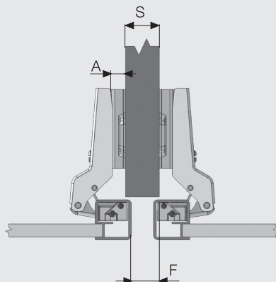
Полунакладные петли
