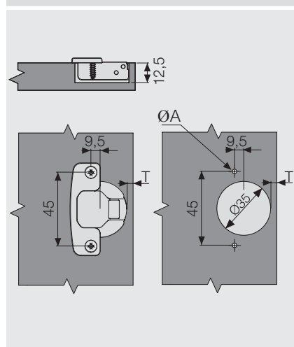
Карта сверления под чашку 45 мм
