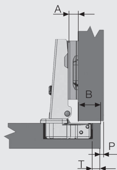
A - Монтажная планка
