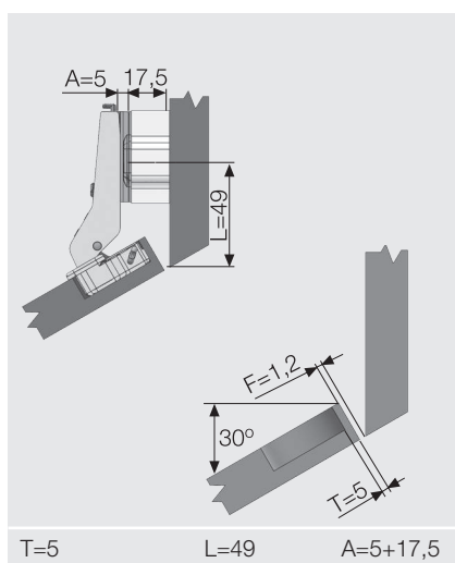
Карта сверления под чашку 45 мм
