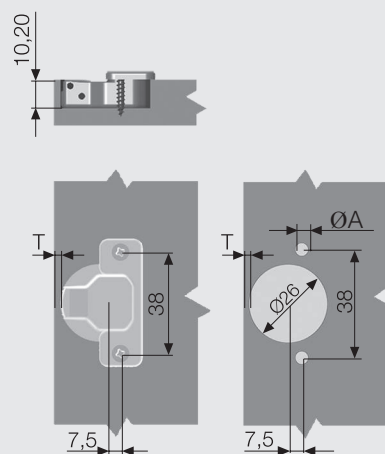
Карта сверления под чашку 38 мм
