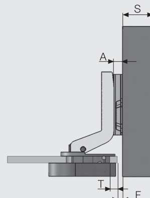
Вкладные петли
