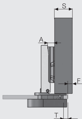
Накладные петли
