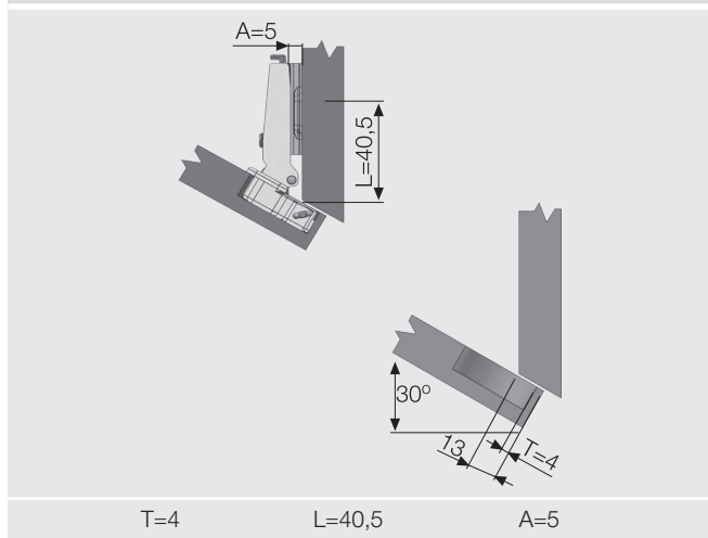
Карта сверления под чашку 45 мм
