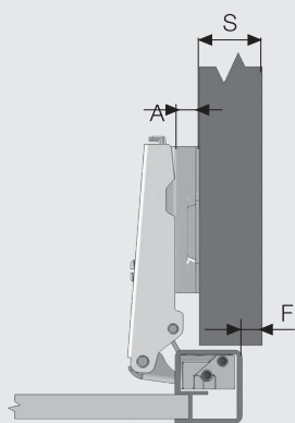
Накладные петли
