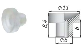
E013 D10
